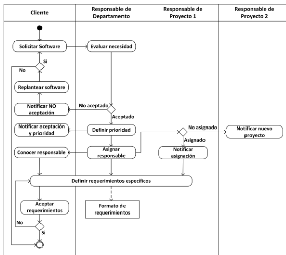
Figura 3. Diagrama de actividad del proceso de solicitud del proyecto.
