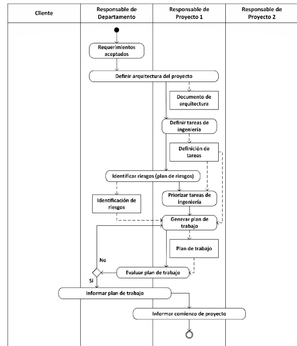
Figura 4. Diagrama de Actividades del proceso de definición del proyecto
